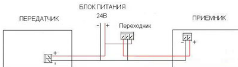
СХЕМА ПОДКЛЮЧЕНИЯ СЧЕТЧИКОВ
